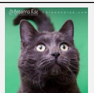
DANTE
